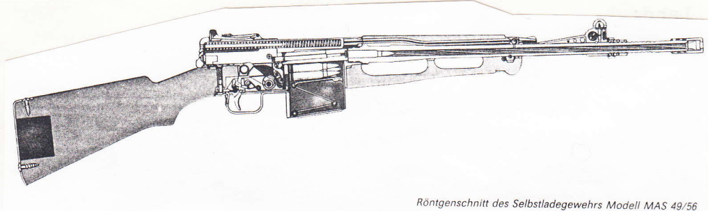
Röntgenschnitt des Selbstladegewehrs Modell MAS 49/56
