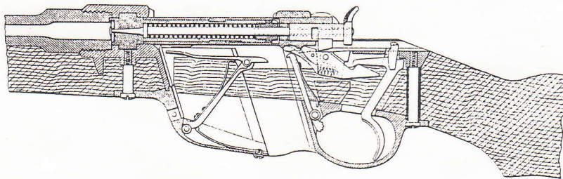
Längenschnitt bei geöffnetem Verschlusse und eingeführtem Packet.
