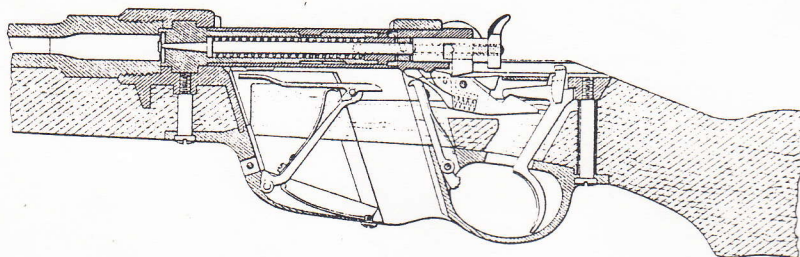
Längenschnitt bei geöffnetem Verschlusse und eingeführtem Packet.
