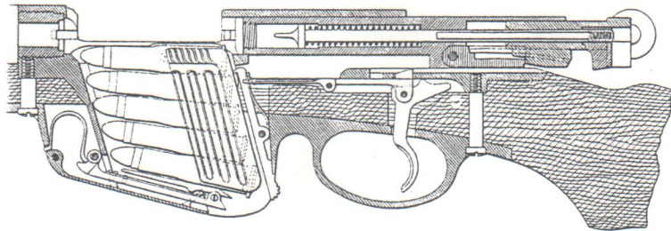
Längenschnitt bei geöffnetem Verschlusse und eingeführtem Packet.
