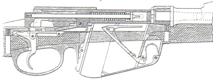
Längenschnitt bei geschlossenem Verschlusse, gespannter Schlagfeder und 5. Patrone geladen.
