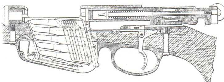
Längenschnitt bei geöffnetem Verschlusse und eingeführtem Packet.
