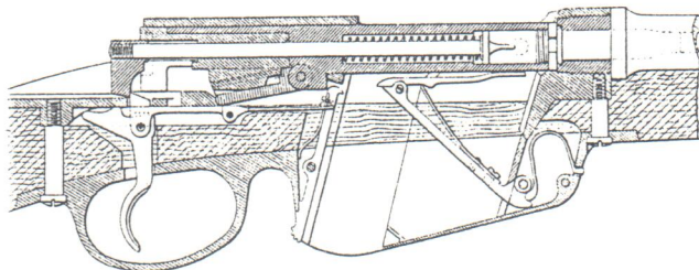
Längenschnitt bei geschlossenem Verschlusse, gespannter Schlagfeder und leerem Kasten.
