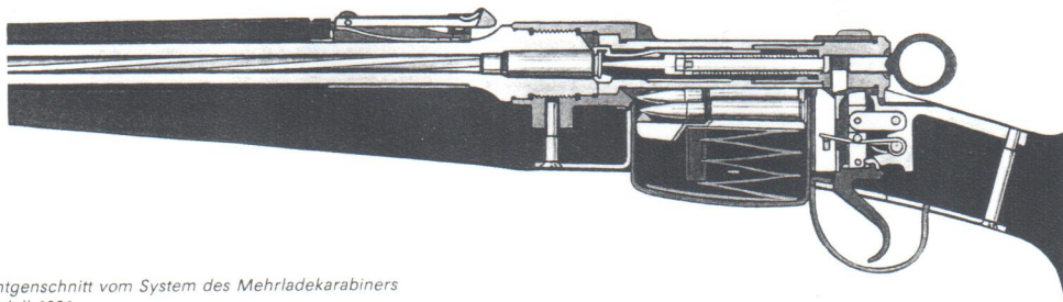
Mehrlade-Scharfschützenkarabiner Modell 1931/43 von rechts
