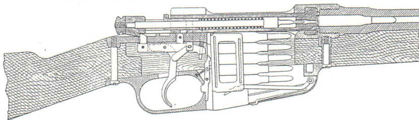
Längenschnitt bei geschlossenem Verschlusse u. gespannter Schlagfeder.
