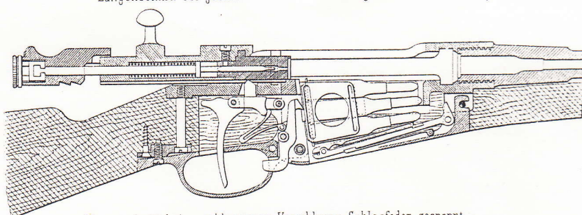
Längenschnitt bei geschlossenem Verschlusse; Schlagfeder gespannt. (1. Patrone abgeschoben).
