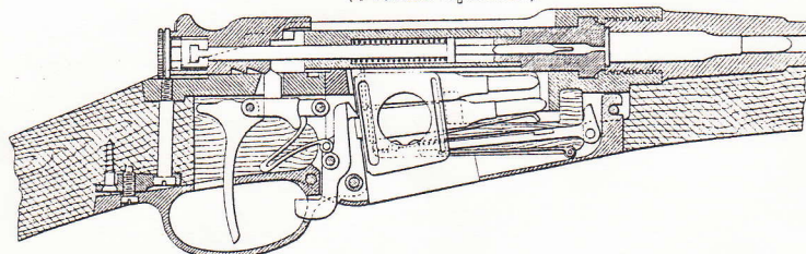
Längenschnitt bei geschlossenem Verschlusse; Schlagfeder gespannt. (1. Patrone abgeschoben).
