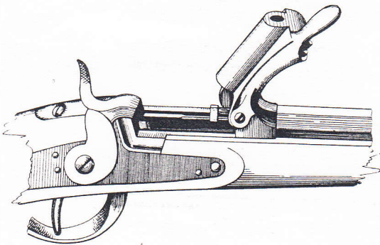
Hinterlader von Wänzl (geöffnet)
