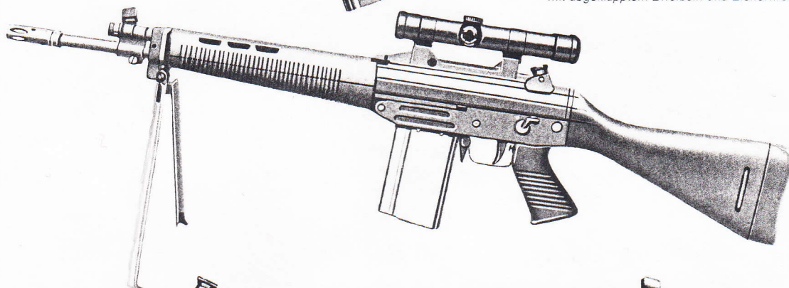
Schnellfeuerwaffe Modell SIG 540 von links mit abgeklapptem Zweibein und Zielfernrohr
