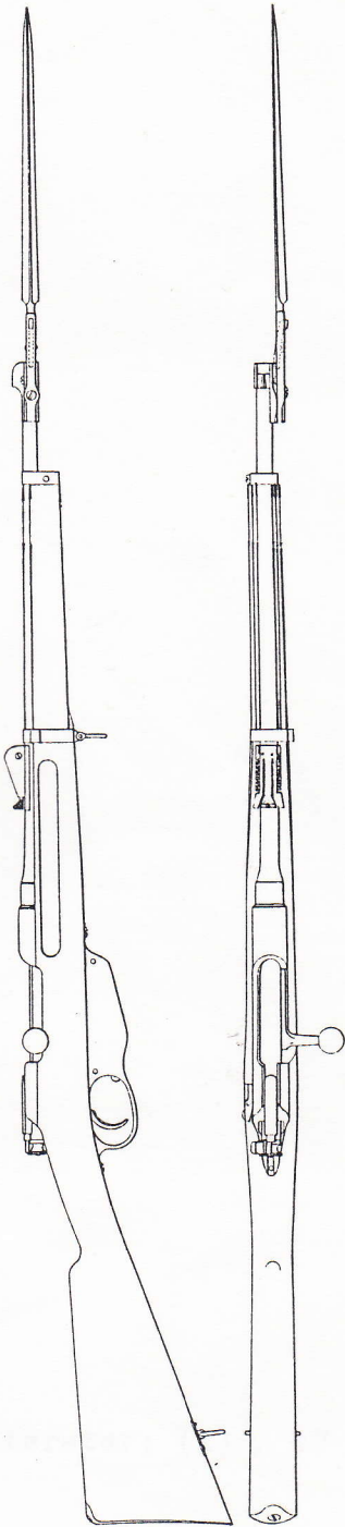
Carabiner mit aufgeklapptem Bajonnet.
