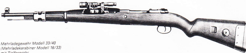
Mehrladegewehr Modell 33/40 (Mehrladekarabiner Modell 16/33) von rechts (mit Kolbenschuh und Schutzblech)
